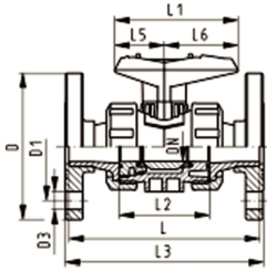
DN10/15 - 50
